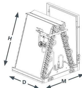
DIMENSIONS DU SERPENTIN EN BOÎTIER (EN POUÇES)
